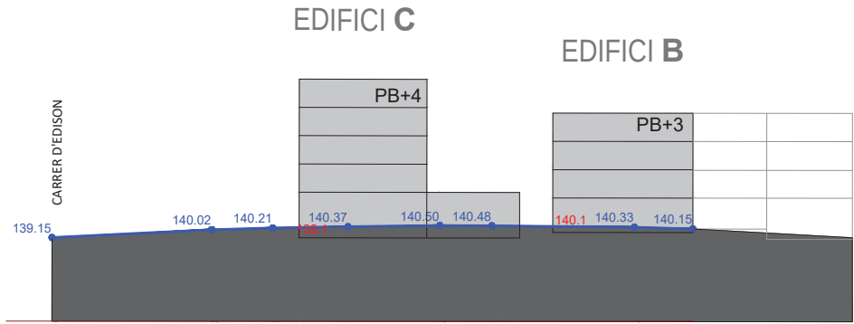
SECCIÓ 2
