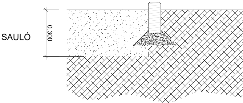
DETALL PAVIMENT DE SAULÓ
