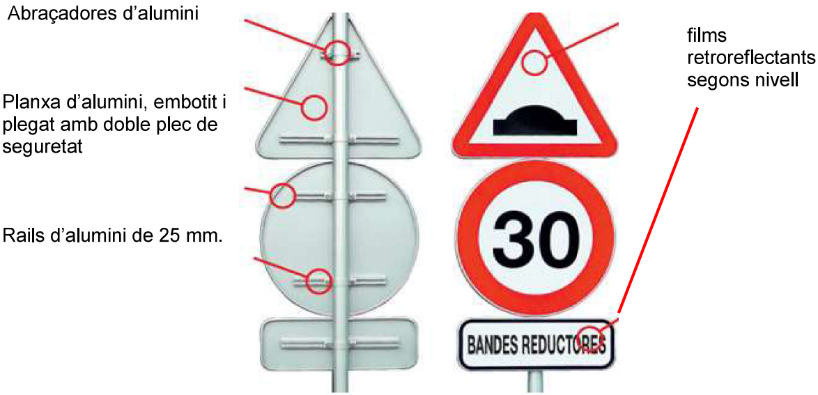
Imatge 1. Model de senyalització i fixació.
