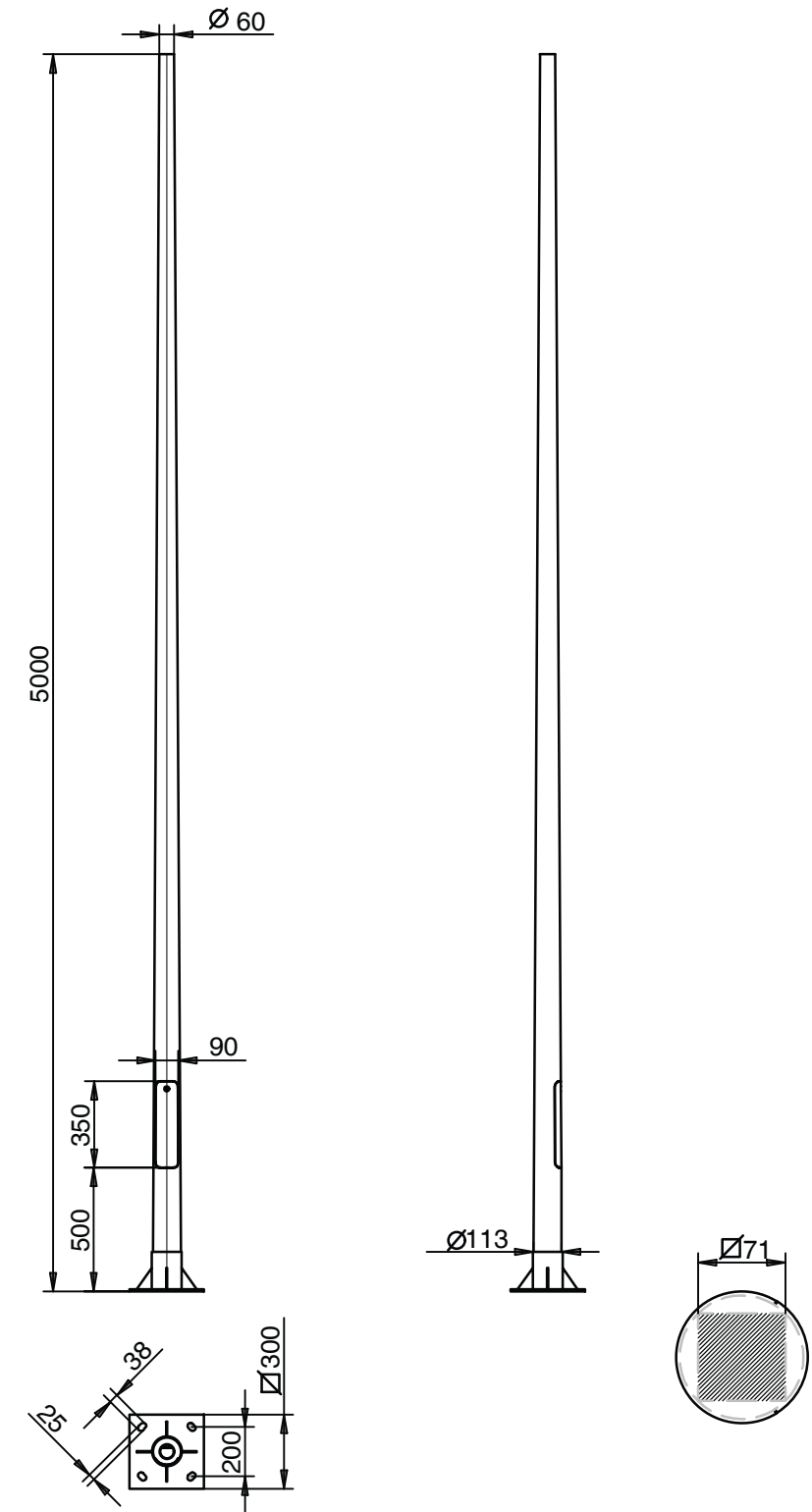
COLUMNA TRONCOCÓNICA 5 M - esc.: 1 / 30
