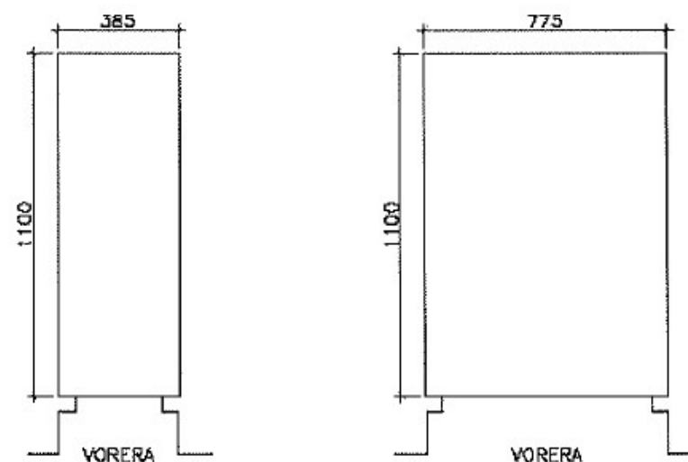
Figura 1 : Armari d'intempèrie TIPUS 1
