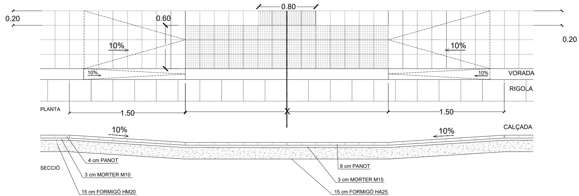
DETALL GUAL DEPRIMIT - esc.: 1 / 30
