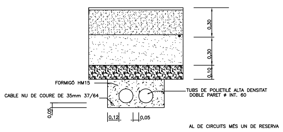
DETALL A-4 RASA TIPUS PER ENTUBAR CABLES A ZONES ENJARDINADES NOTA: ES COL·LOCARÀ IN NOMBRE DE TUBS IGUAL AL DE CIRCUITS MÉS UN DE RESERVA
